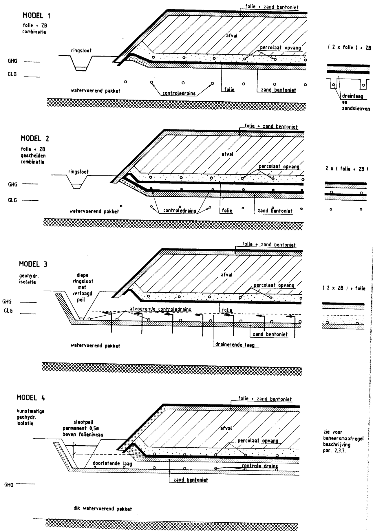
figuur 4 Onderafdichtingsconstructies
